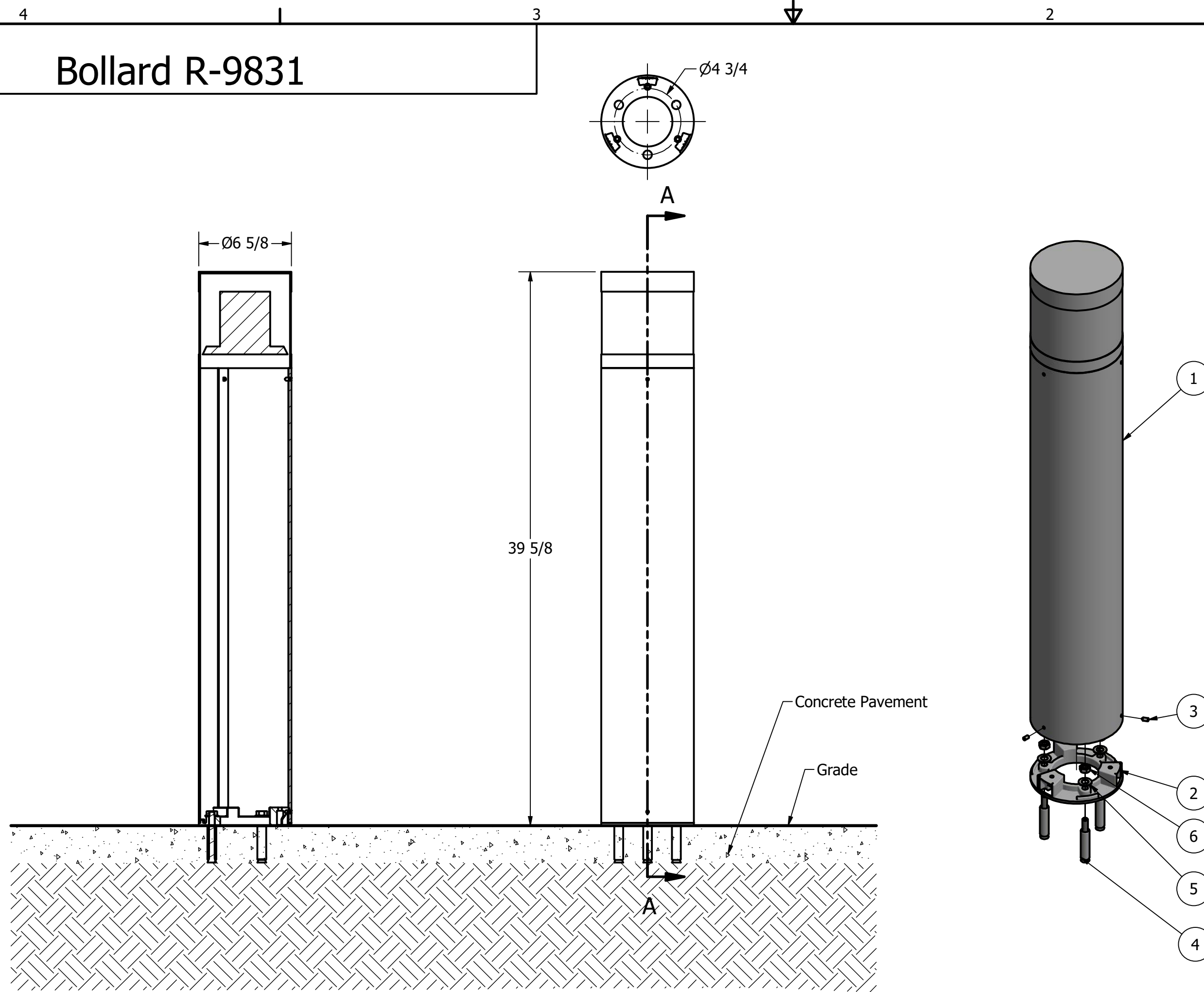
SECTION A-A
