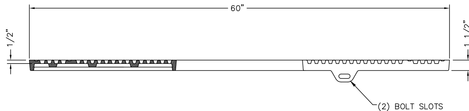
SECTION A-A
