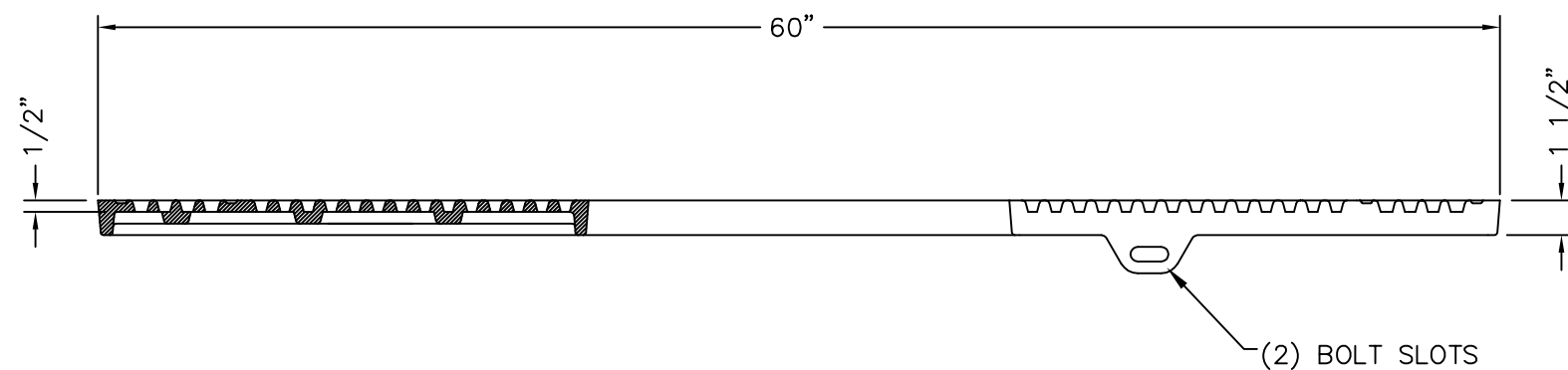
SECTION A-A
