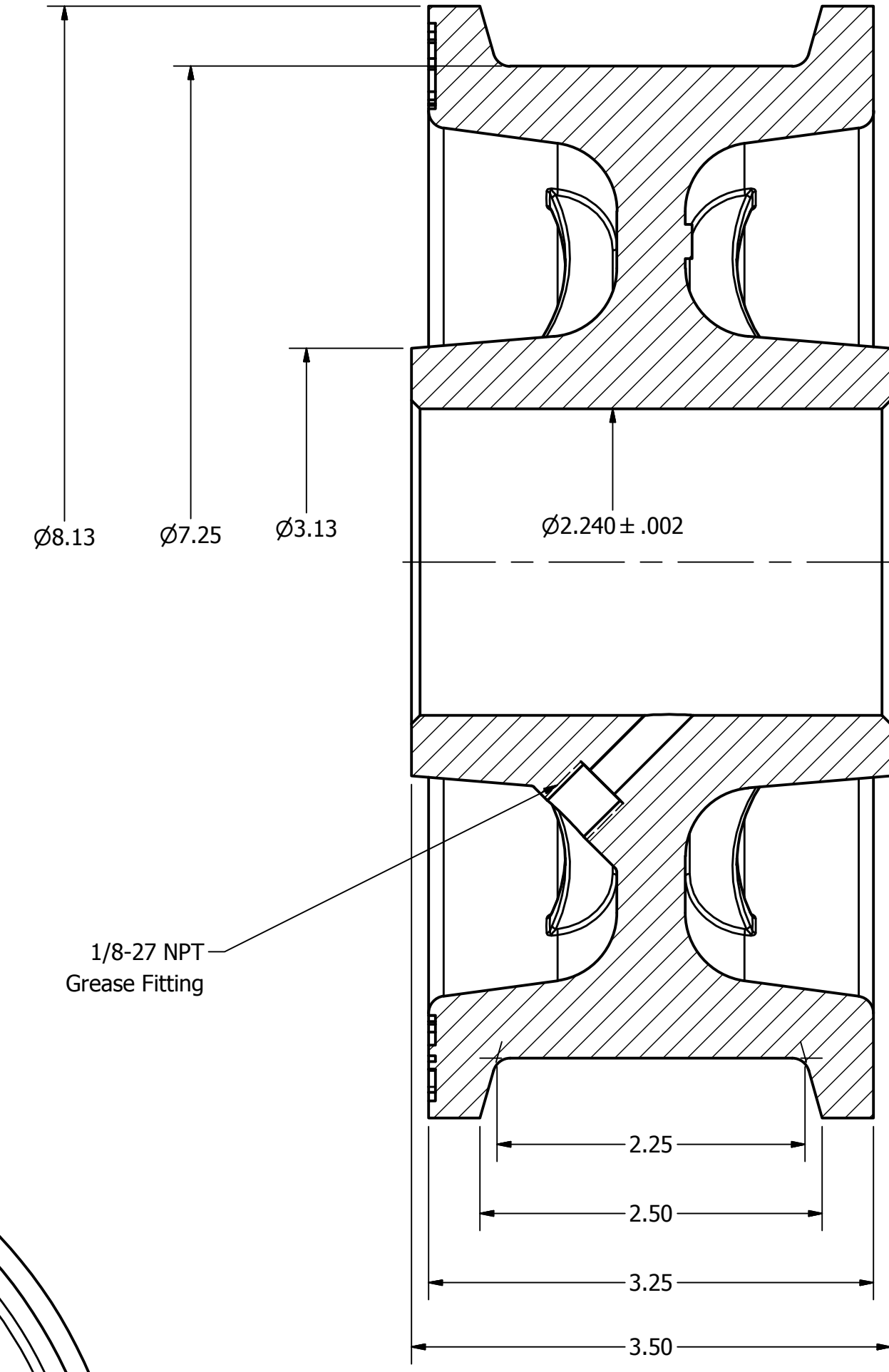
SECTION A-A
