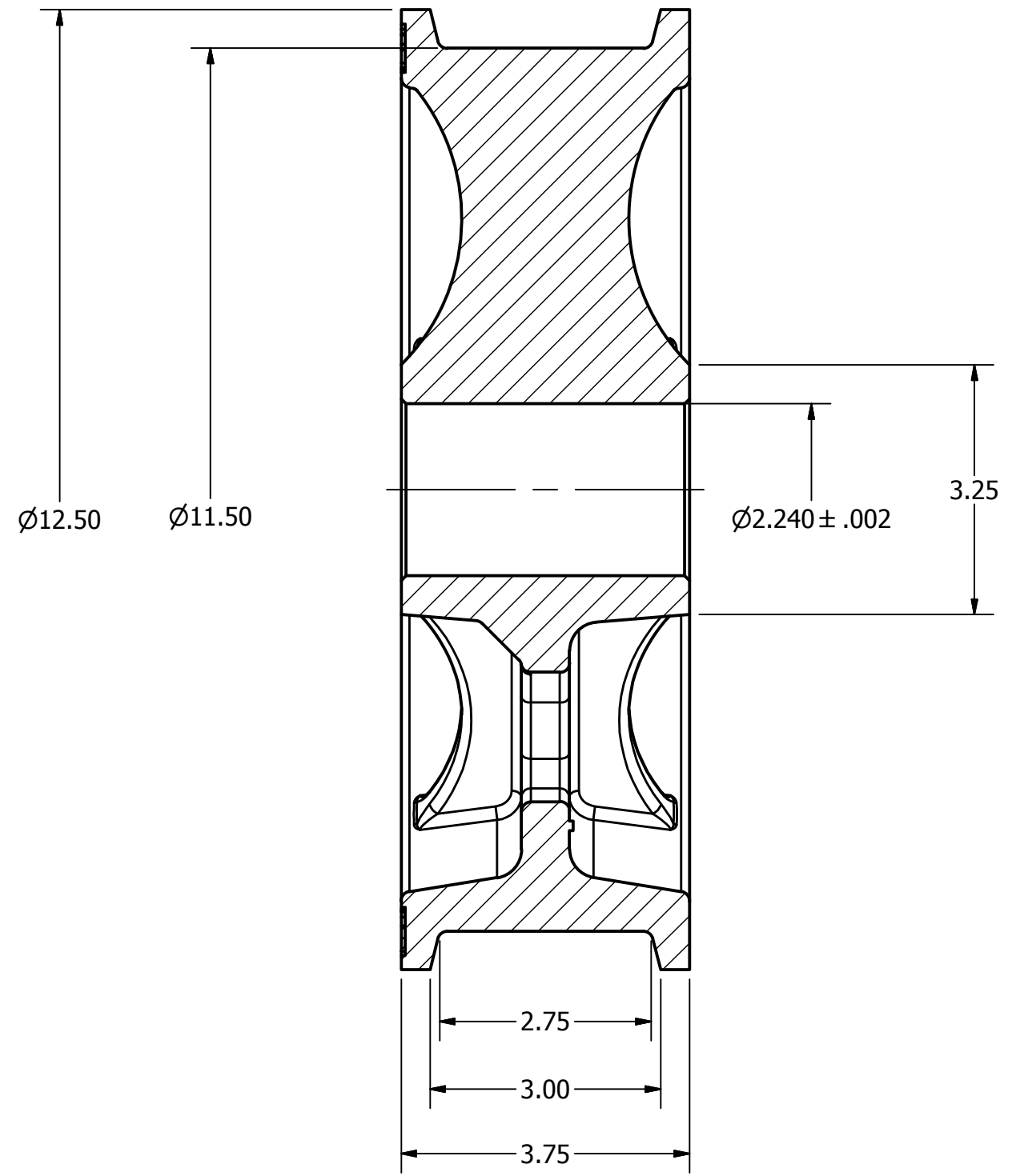
SECTION A-A
