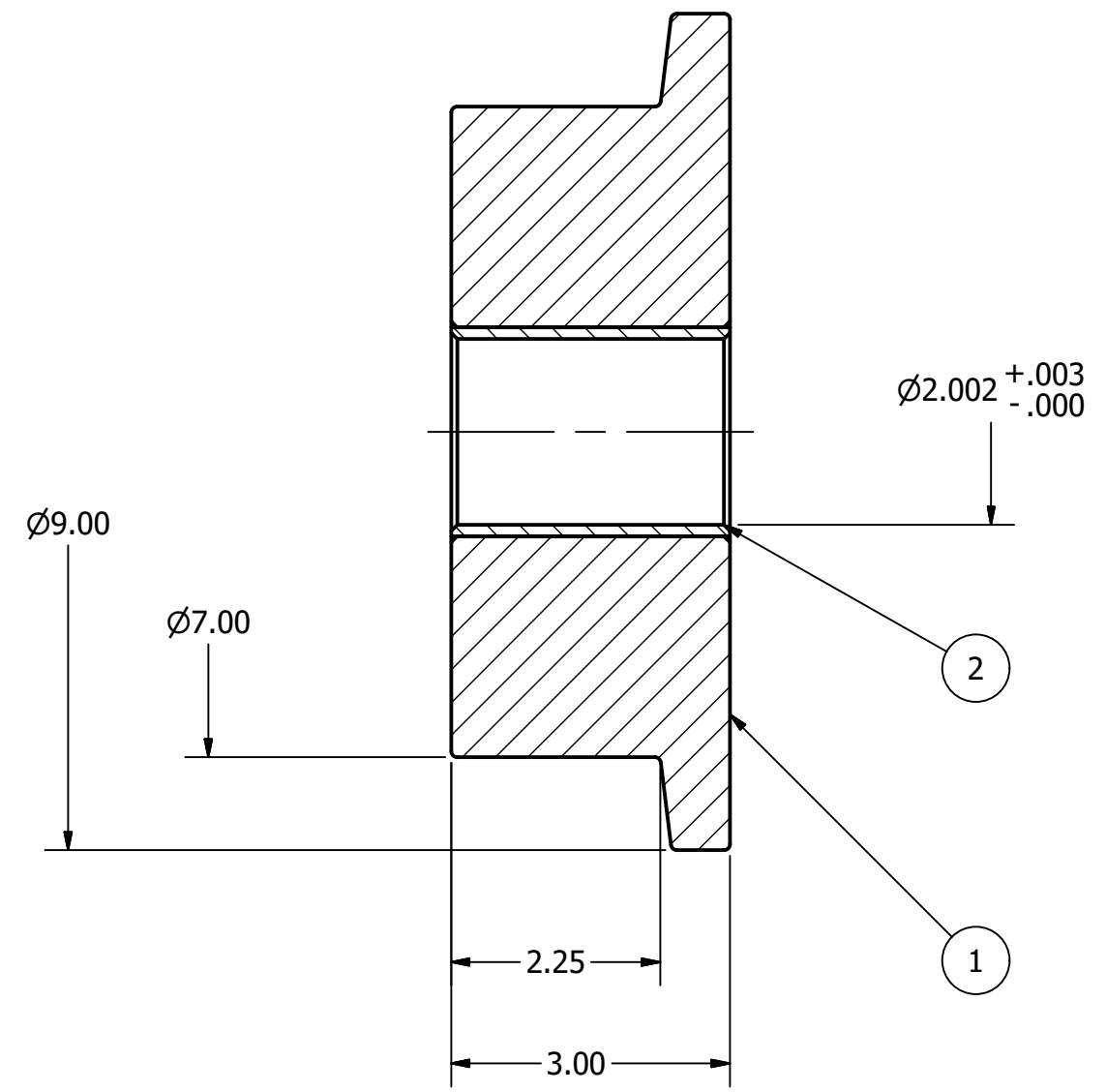
SECTION A-A
